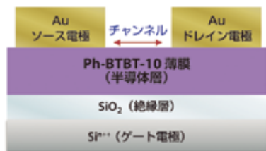
図 1. OFET 素子構造
