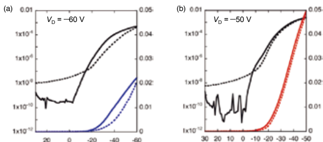
図 2. 蒸着型 OFET 素子の伝達特性
