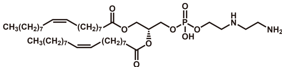
DOP-DEDA
