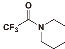
1-(Trifluoroacetyl)- piperidine 5g 8,100円 / 25g 27,200円 [T2087]
