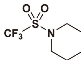
1-(Trifluoromethanesulfonyl)- piperidine 5g 11,900円 / 25g 41,500円 [T4342] New
