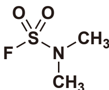
Dimethylsulfamoyl Fluoride 5g 12,000円 / 25g 41,800円 [D6323] New
