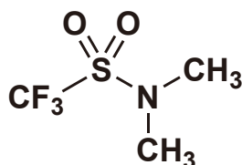
N,N-Dimethyl- trifluoromethanesulfonamide 1g 4,300円 / 5g 14,800円 / 25g 51,800円 [D6135] New
