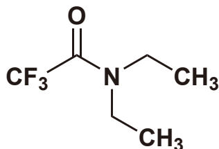
N,N-Diethyl- 2,2,2-trifluoroacetamide 5g 9,100円 / 25g 32,000円 [D5063]
