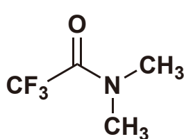
2,2,2-Trifluoro- N,N-dimethylacetamide 5g 6,000円 / 25g 18,100円 [T3262]
