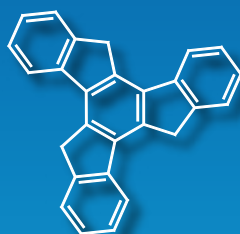
Truxene
