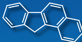
1,2-Benzofluorene
