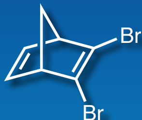
2,3-Dibromonorbornadiene
