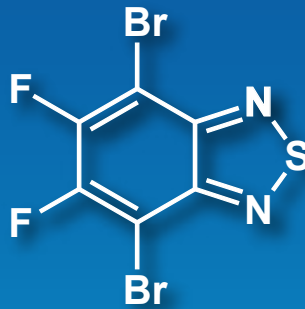
4,7-Dibromo-5,6-difluoro- 2,1,3-benzothiadiazole
