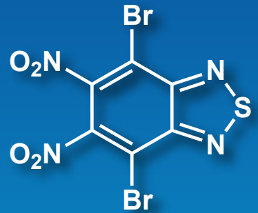
4,7-Dibromo-5,6-dinitro- 2,1,3-benzothiadiazole
