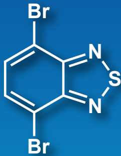
4,7-Dibromo- 2,1,3-benzothiadiazole
