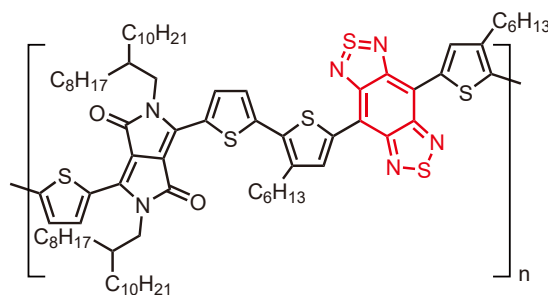
PBBT6-DPP 5)
