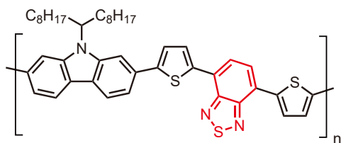
PCDTBT 4)
