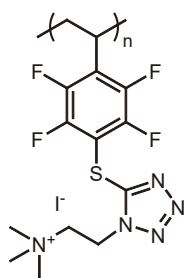
レドックスフロー電池 陰イオン交換膜 1)
