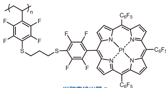
光酸素検出膜 3)
